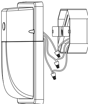
✖ 3. Connect wire
